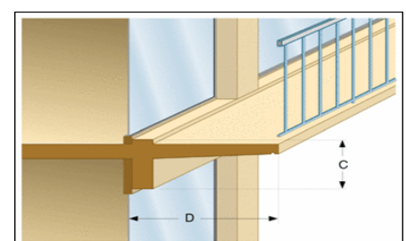
La règle C+D
